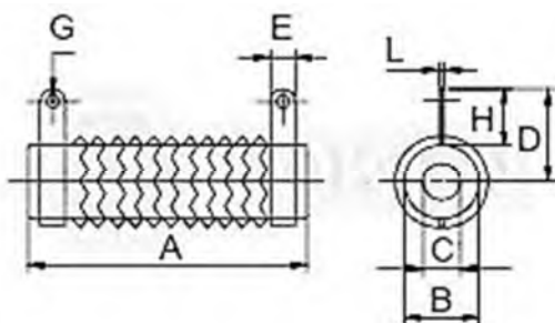
(DQ-A) N - No Mount
