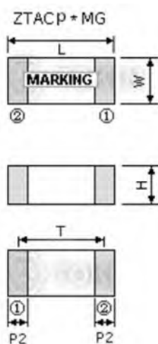
MHz (ZTACP*MG) Dimensions
