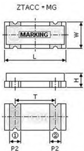
MHz (ZTACC*MG) Dimensions
