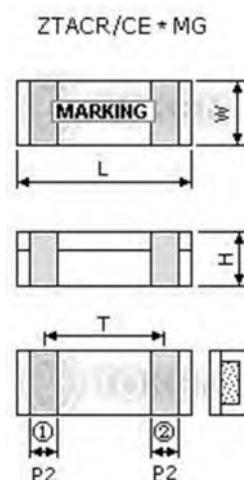
MHz (ZTACR/CE*MG) Dimensions
