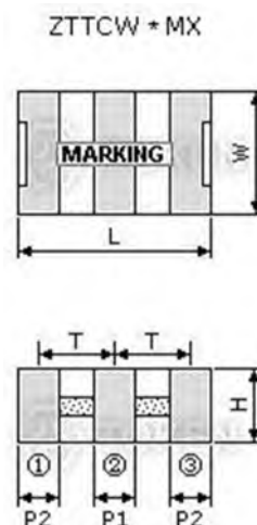
MHz (ZTCS/CV*MT/MX) Dimensions
