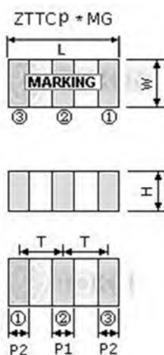
MHz (ZTTC*MG) Dimensions
