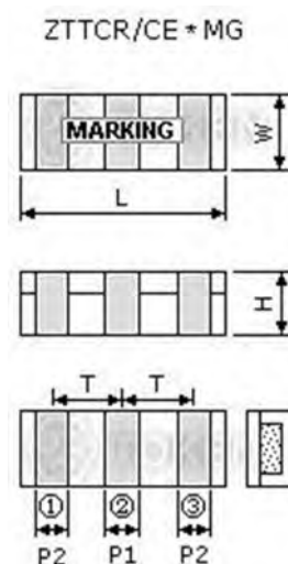
MHz (ZTTCR/CE*MG) Dimensions
