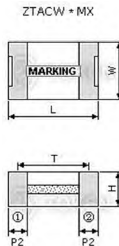
MHz (ZTACS/CV*MT/MX) Dimensions
