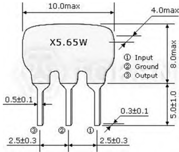
陶瓷陷波器双吸收型 XT MW 系列 尺寸图
