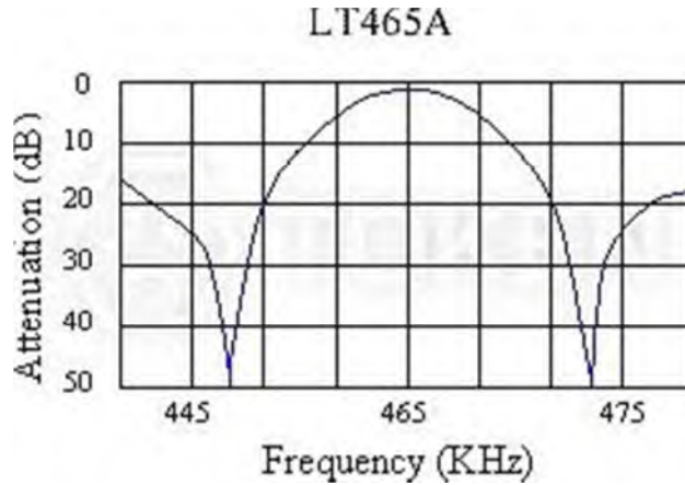
LT 收录机用系列 特性曲线
