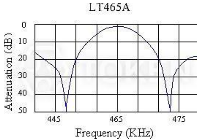
LT 收录机用系列 特性曲线
