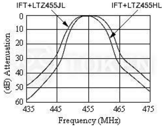
LTZ 系列 - 特性曲线
