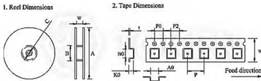
贴片电感线圈盘及编带尺寸 (单位: mm)
