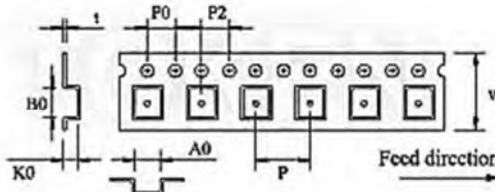
贴片电感线圈盘及编带尺寸 (单位: mm)
