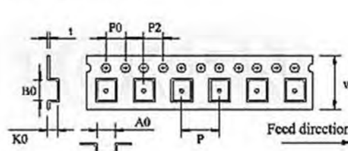
贴片电感线圈盘及编带尺寸 (单位: mm)
