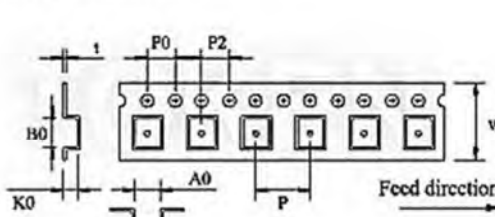
贴片电感线圈盘及编带尺寸 (单位: mm)
